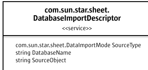
DatabaseImportDescriptor
